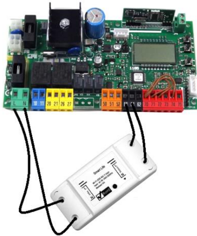
Pav. 4 Pajungimo schema automatikoje
