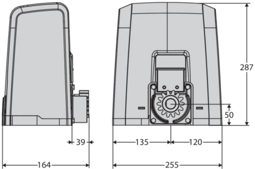
3 pav. Vartų automatika
